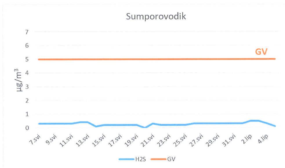
Slika 4.1.2: Kretanje srednjih dnevnih koncentracija sumporovodika ( \mu\text{g}/\text{m}^3 )
