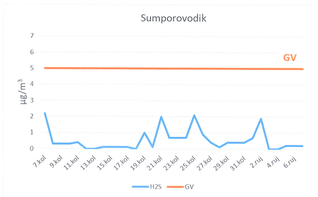
Slika 4.1.2: Kretanje srednjih dnevnih koncentracija sumporovodika ( \mu\text{g}/\text{m}^3 )
