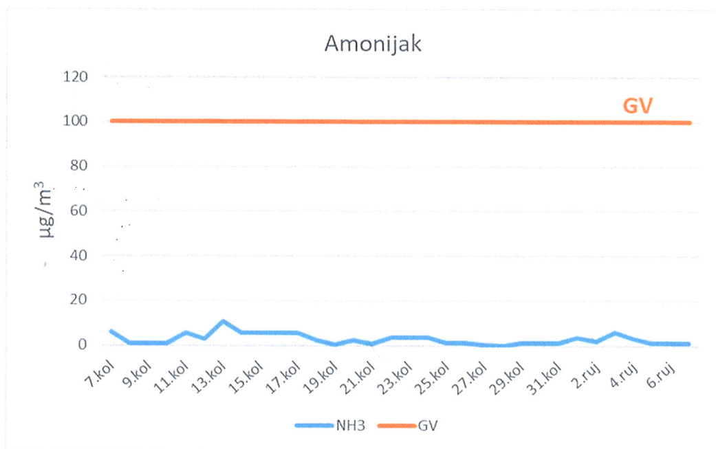
Slika 4.1.1: Kretanje srednjih dnevnih koncentracija amonijaka ( \mu\text{g}/\text{m}^3 )
